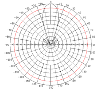
H-Plane
